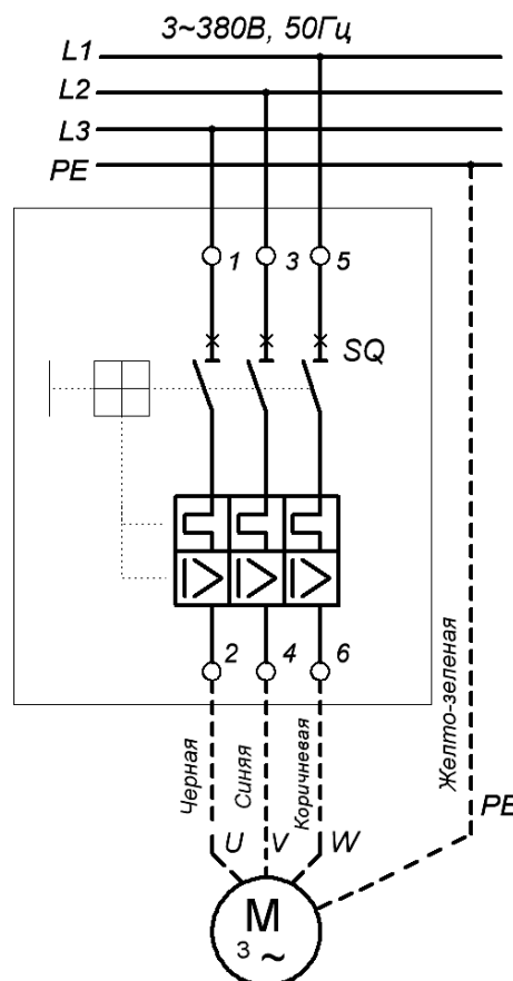
Рисунок 7 – Схема подключения
